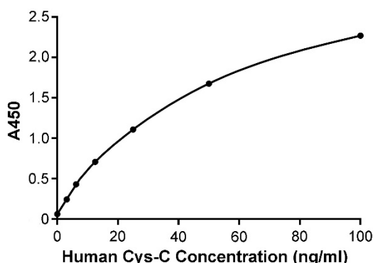
图3. Human Cys-C ELISA Kit的标准曲线。实测数据会因实验条件、检测仪器等的不同而存在差异，图中数据仅供参考。
